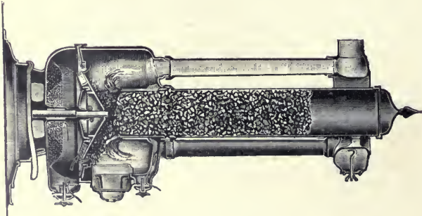
14. ábra. Feyér-féle barnaszénkályha.
