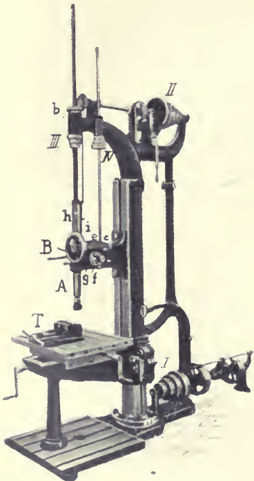
3. ábra. Oszlopos fúrógép.
