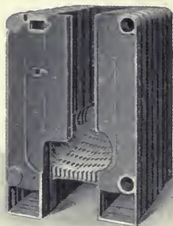
Körting-féle kazán nyitott tagsora.
