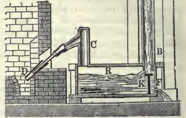
4. ábra. Hidraulikus fuvógép.
