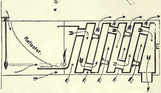
2. ábra. Szekrényes gázkályha a Révai-téle egyarából.
