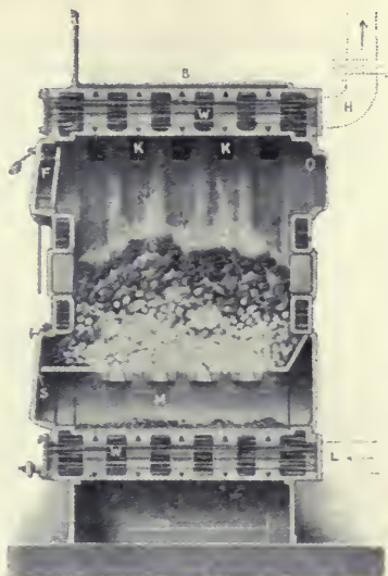
Strebelt-féle vízkazán hosszsmetszete.
