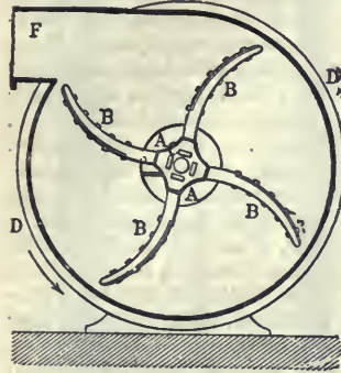
6. ábra. Körforgású centrifugális ventilátor.
