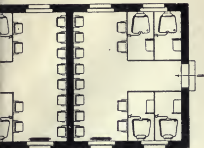
4. sz. ábra. Munkásfürdő alaprajza 8 zuhanyfülkével és 24 mosdóval.
