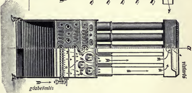
3. ábra. Oszvos gázkályha.
