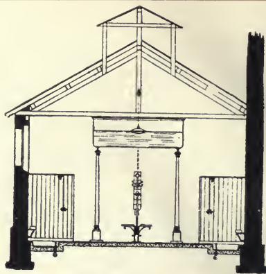
2. sz. ábra. Munkásfürdő metszete melegvízmedencével, öltözőpadokkal és zuhanyílkékkel.
