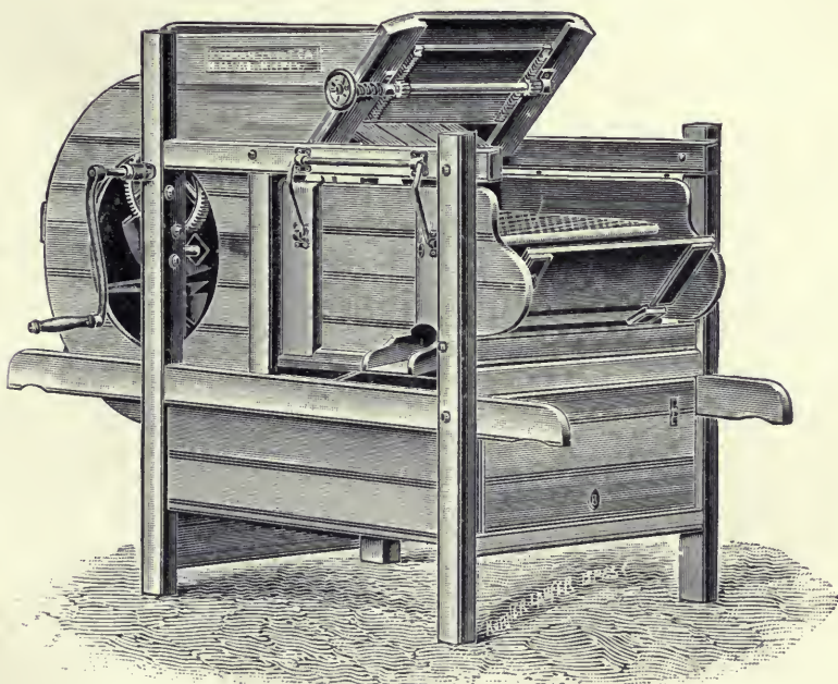
Kalmár-féle gabonarosta.
