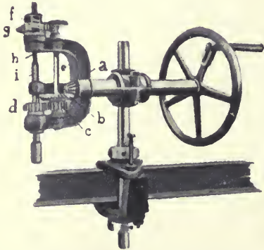
2. ábra. Kézzel hajtott fúrógép.
