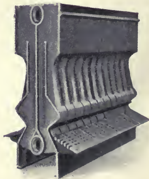
Catena-kazán közbelső tagsora.
