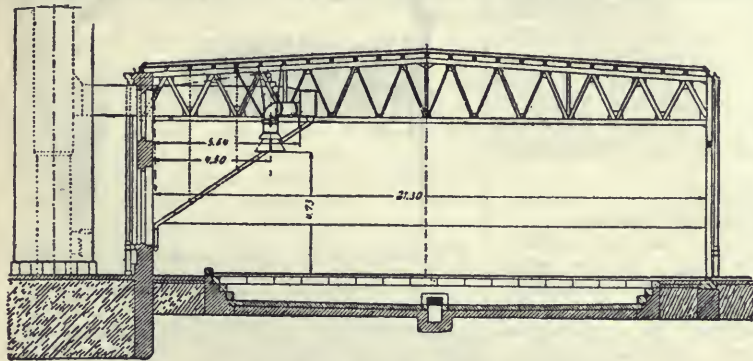
8. ábra. Gyűrlőalakú fűtőház fűstelvezető csatornával.
