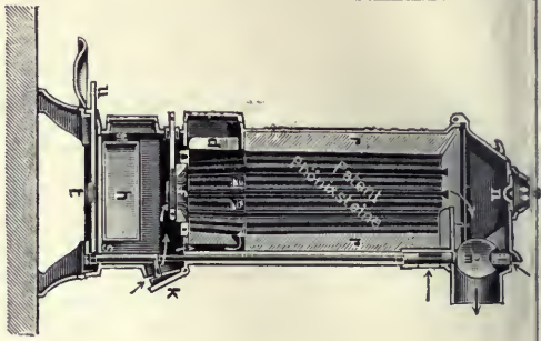
6. ábra. Tűlkályha tisztító belsősele.
