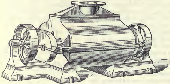
3. ábra. Roots-Blower. A gép külseje.
