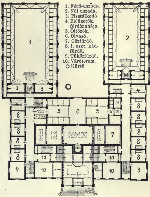
5. sz. ábra. A kölni Hohenstaufen-fürdő fsz. alaprajza.
