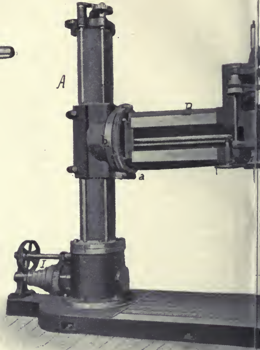
4. ábra. Egyetemes sugárfúrógép.
