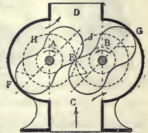
2. ábra. Root-féle fuvó keresztmetszete (Roots-Blower).
