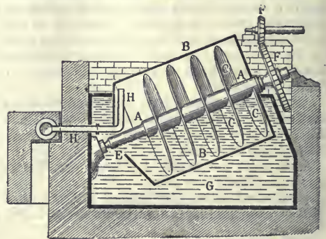
5. ábra. Csavarfuvó (cagniardelle).
