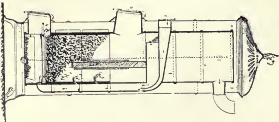
13. ábra. Izard-féle barnaszénkályha.
