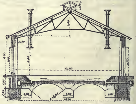
7. ábra. Gyűrűalakú fűtőház metszete.
