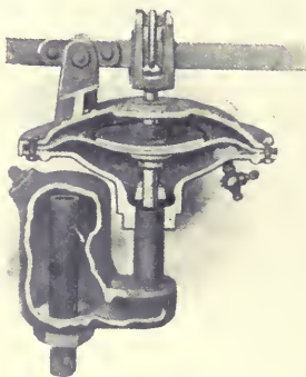
Membrános égésszabályozó gőzkazánokra.
