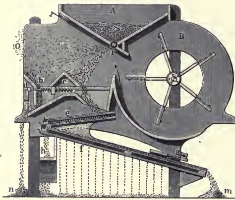
Tarár, rostával egyesítve.
