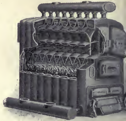
Vízszintes füstforgatású öntöttvas kazán.
