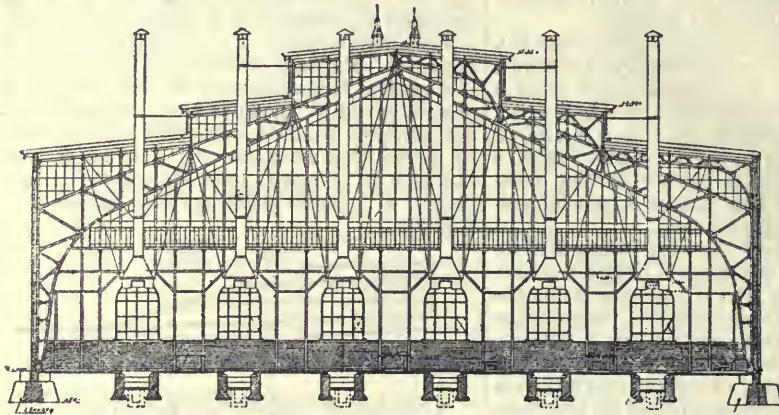
3. ábra. Négyoszlopalakú fűtőház metszete.
