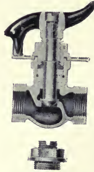
Elzáró- és szabályozó-szelep.
