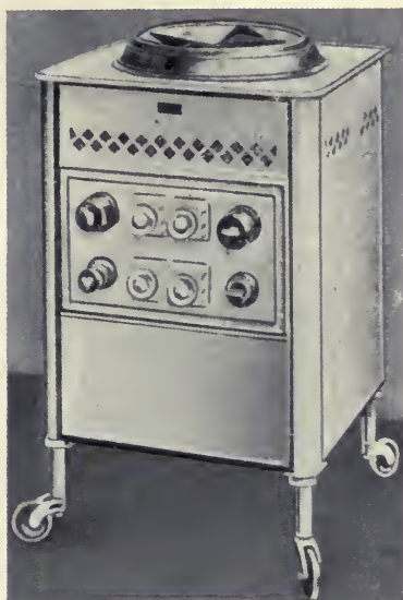
A Siemens-Schuckert cég hordozható ózon-ventilátora.
