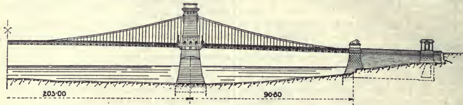
1. ábra. A budapesti lánchíd hosszmetsete.
