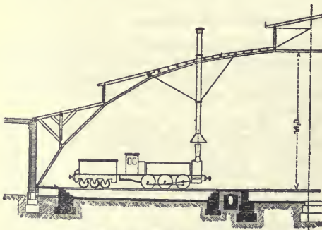
5. ábra. Körűfűtőház metszete.
