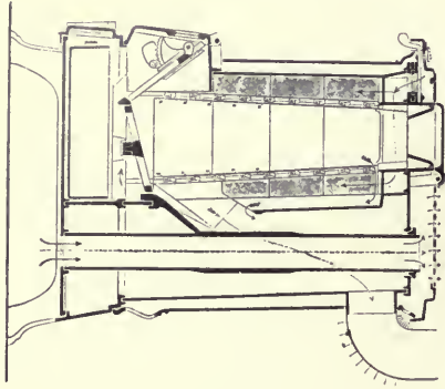
11. ábra. «Perpetuum»-kályha.
