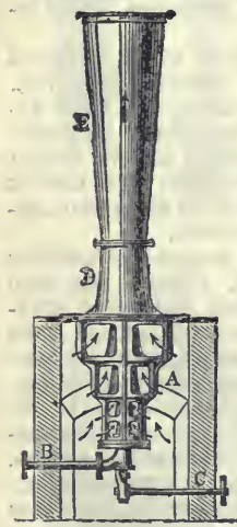
7. ábra. Körting gőzsugár-ventilátora.
