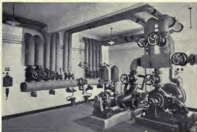
Távfűtő-berendezés szivattyu- és főgőzelosztó állomása.
