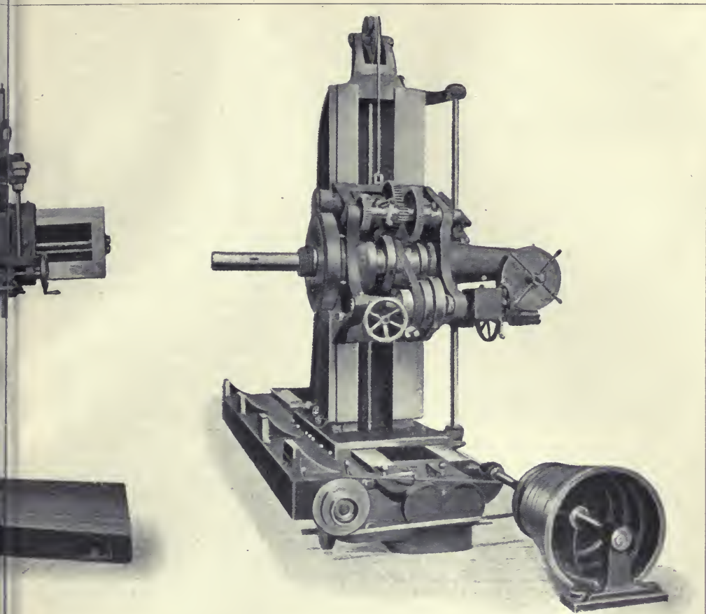
6. ábra. Vízszintesen fűrő gép elmozdítható főorsóval, nagy öntvények fúrására.
