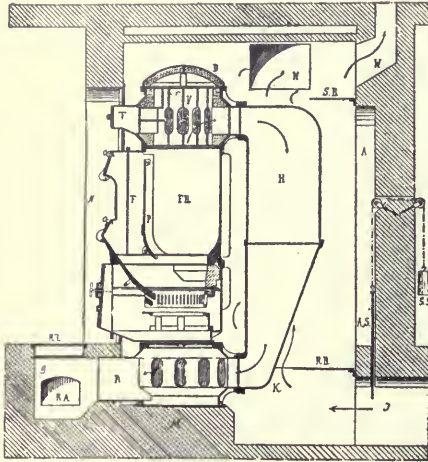
Kori-féle kalorifer metszete.
