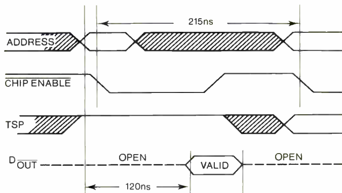
4K MOS RAM
